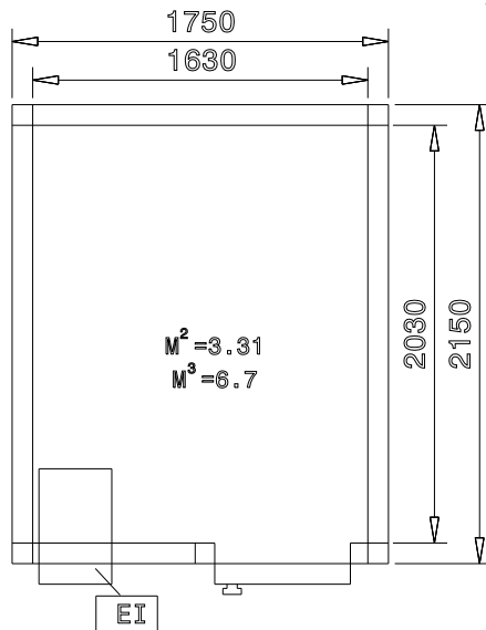
Boven aanzicht
